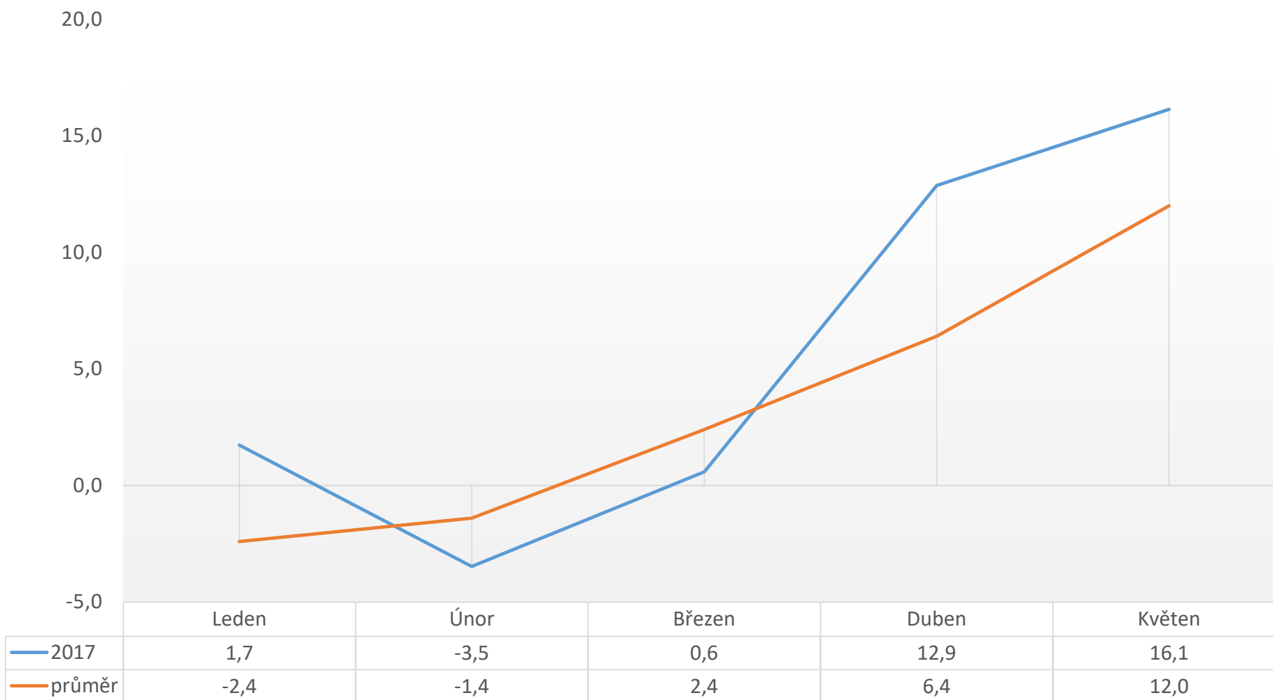
Teploty 2018
