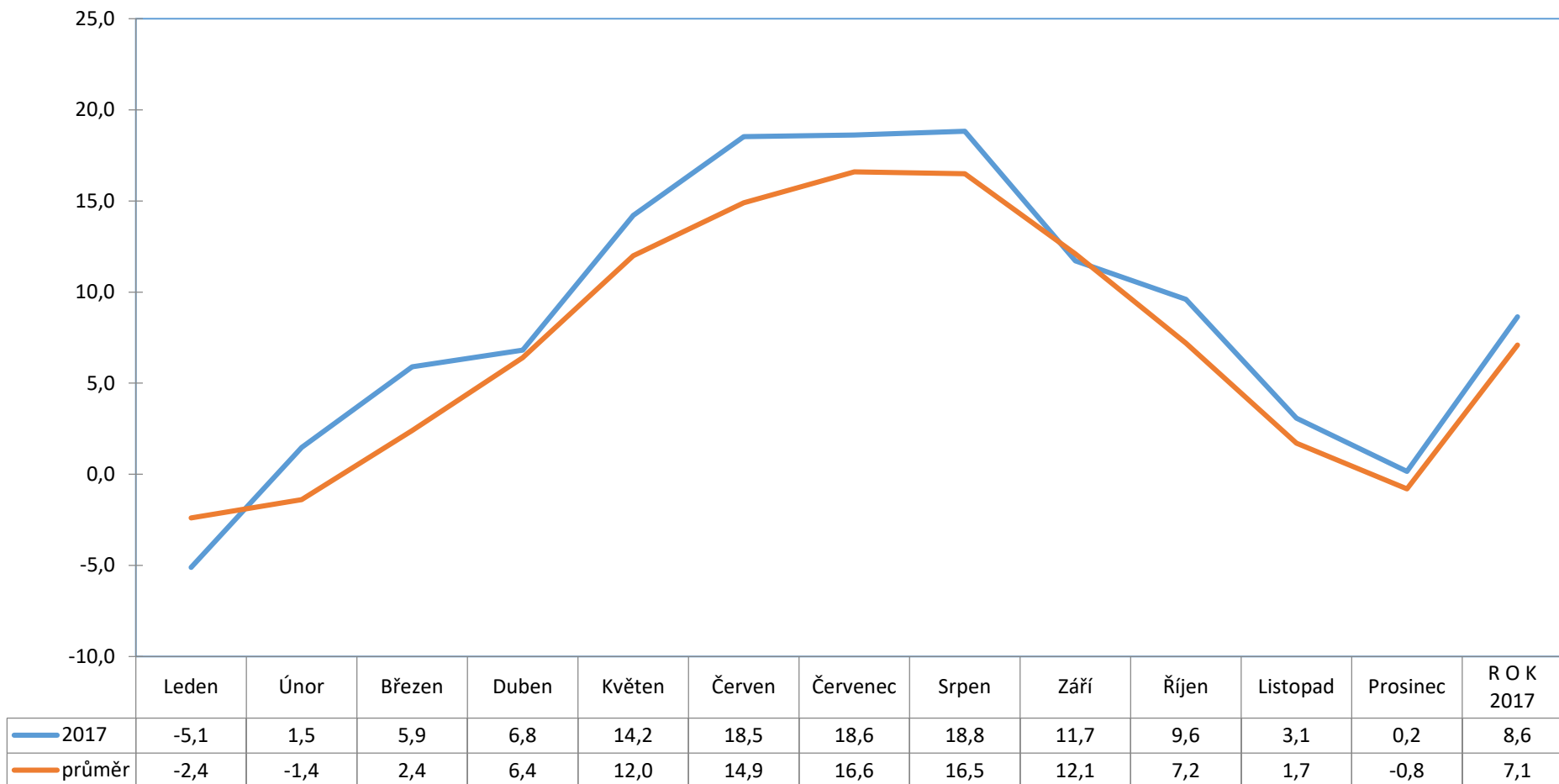
Průběh teplot 2017
