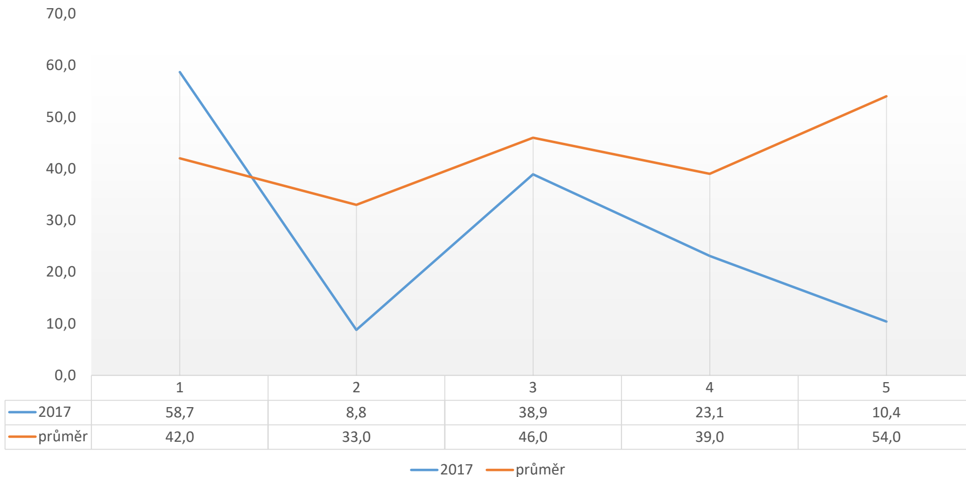
Srážky 2018
